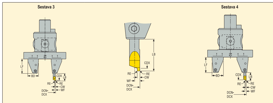
Tabulka pro výběr: nástroj pro čelní zápichy – ve dně otvoru s MPA adaptérem, pro hlavy EPB 760
