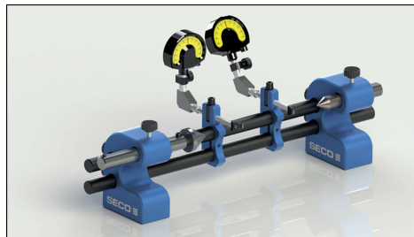
SF-60200-C160C190: produkt. číslo 02885396
