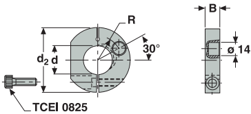
Kroužek pro přívod chladičí kapaliny
