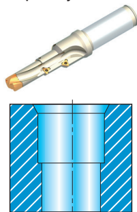
B2. Dva průměry a sražení hrany
