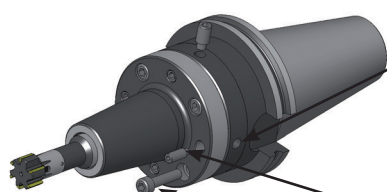
Radiální stavěcí šrouby (4 kusy)
