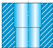
B4. Stupňovitý se sražením hrany
