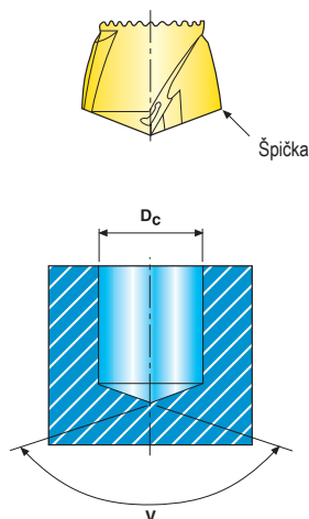
A1. Jeden průměr
