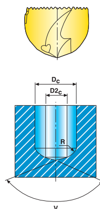
B4. Rádiusový přechod
