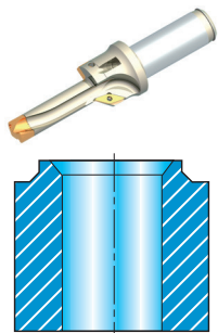
A5. Orovnání a sražení hrany
