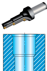
B4. Stupňovitý se sražením hrany
