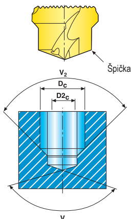
B3. Dva průměry
