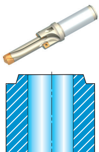
A4. Orovnání čela
