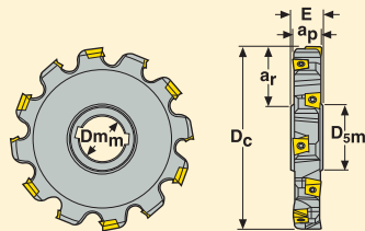
Typ A - plochý – pevná lůžka (Typ A FP)
