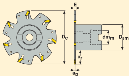
Typ B 3 s unašečem
