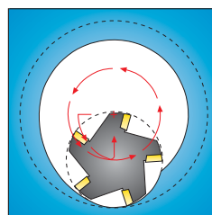
Postupný nájezd do materiálu – doporučená metoda.
