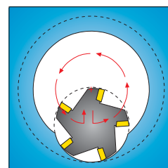
Postupný nájezd do materiálu – snižte posuv na zub.
