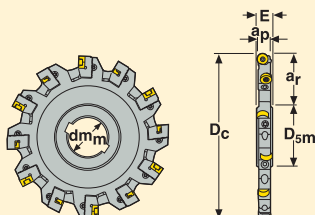
Typ B - s unašečem
