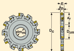
Typ B - s unašečem
