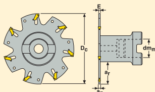
Typ B 2 s unašečem
