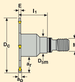
Typ B 4 pro Combimaster
