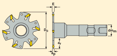
Typ B 1 - válcová/Weldon stopka
