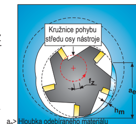
Postupný nájezd do materiálu – snižte posuv na zub.
